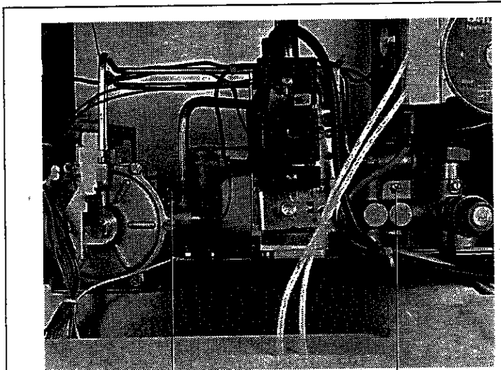
Befestigungsschrauben Wasser-Wasser-Austauscher Viti di fissaggio scambiatore acqua-acqua Foto 10
